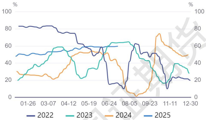
高炉开工率:全国(样本数247家):当周值
